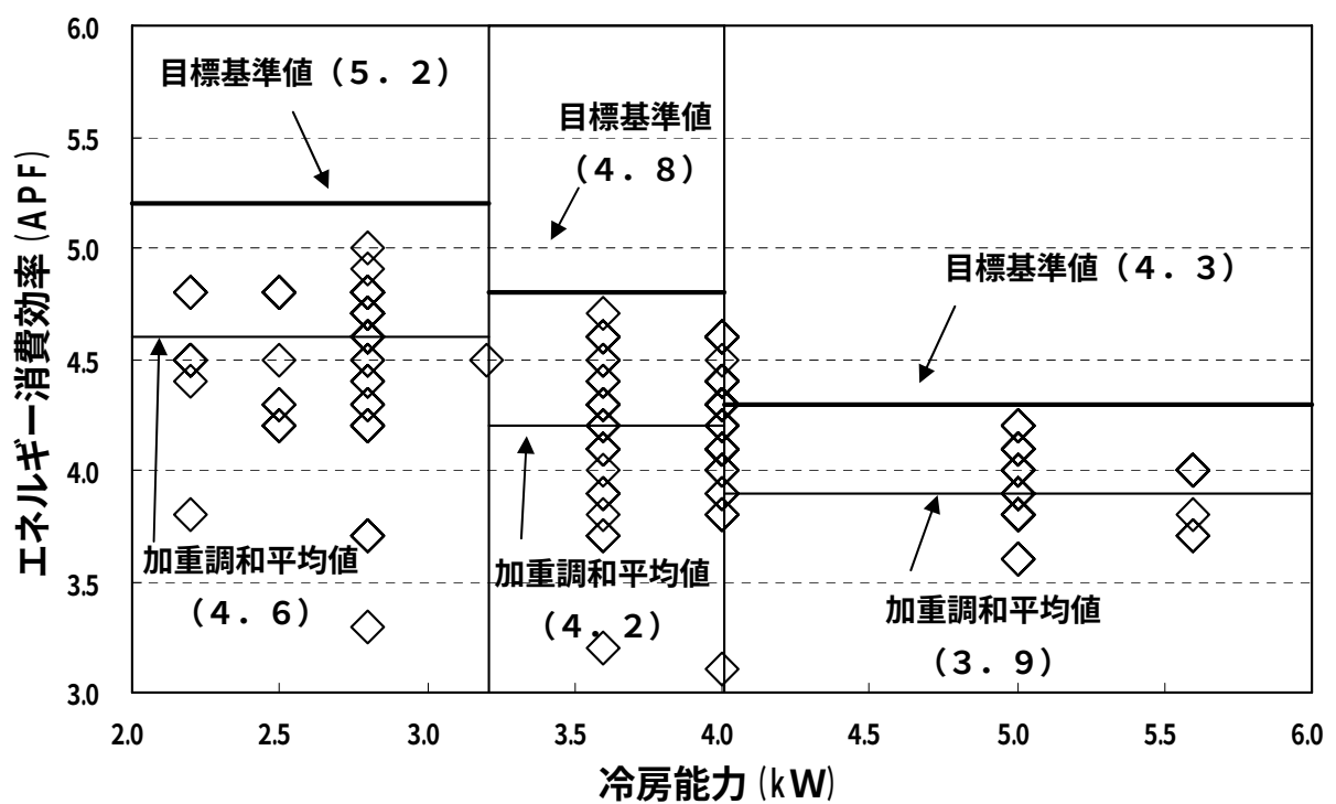
図２．直吹き壁掛け以外の分離形のもののトップランナー値及び目標基準値
