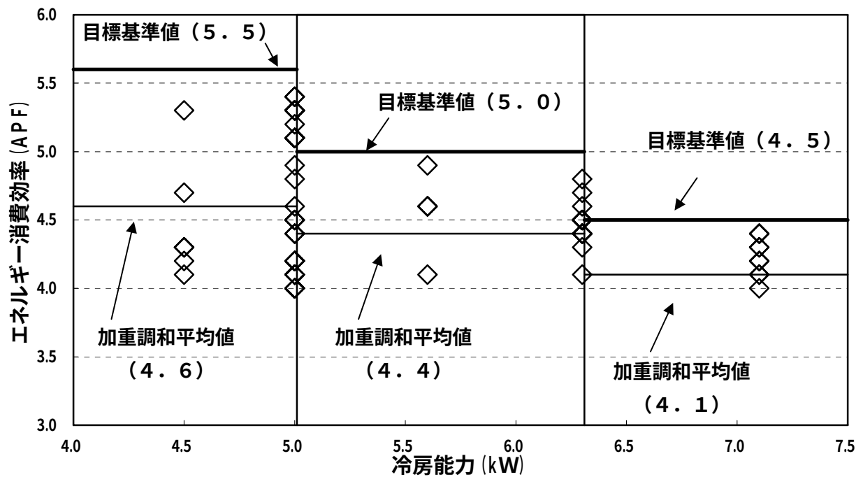
図１．直吹き壁掛けのもののトップランナー値及び目標基準値
