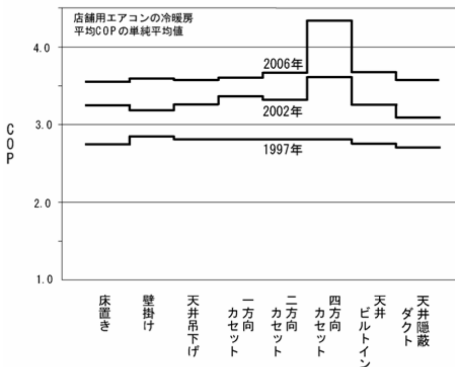
室内機形態別の冷暖房平均COPの推移
