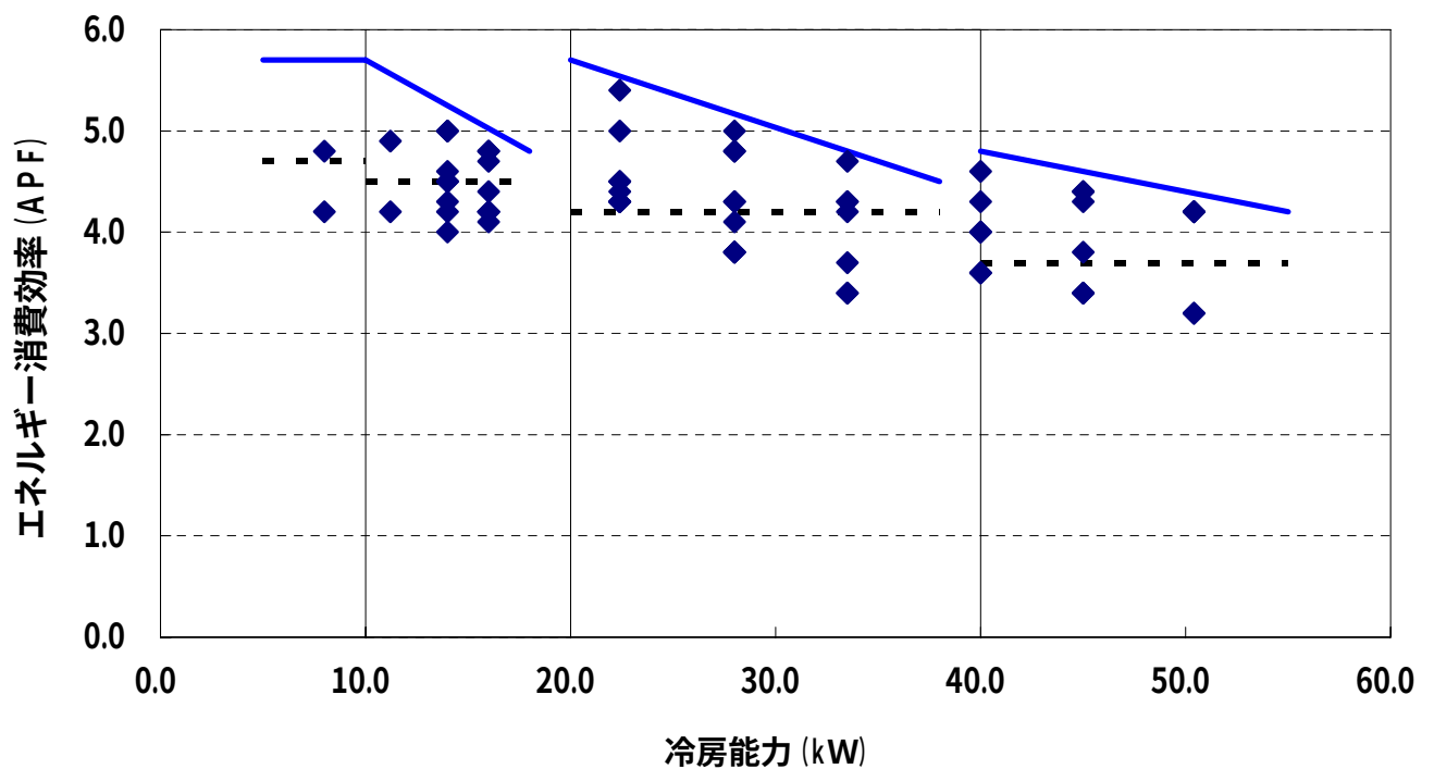
図 9 . ビル用マルチエアコンの目標基準値について
